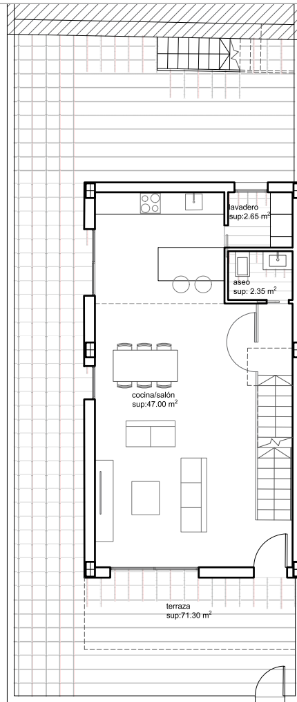
PLANTA BAJA
