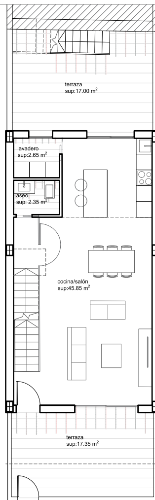
PLANTA BAJA
