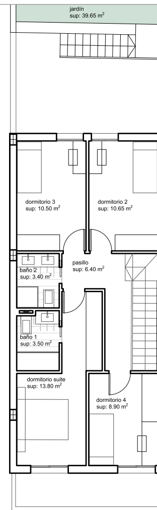
PLANTA PRIMERA
