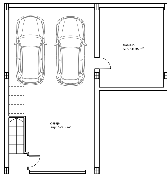
PLANTA SÓTANO
