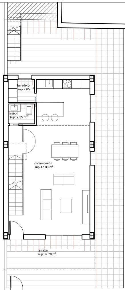
PLANTA BAJA
