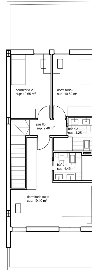
PLANTA PRIMERA
