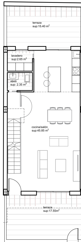
PLANTA BAJA
