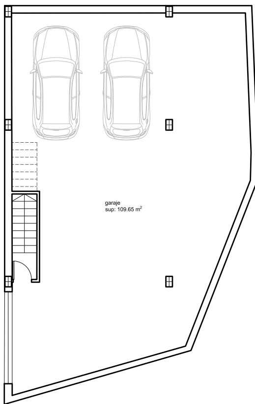
PLANTA SÓTANO
